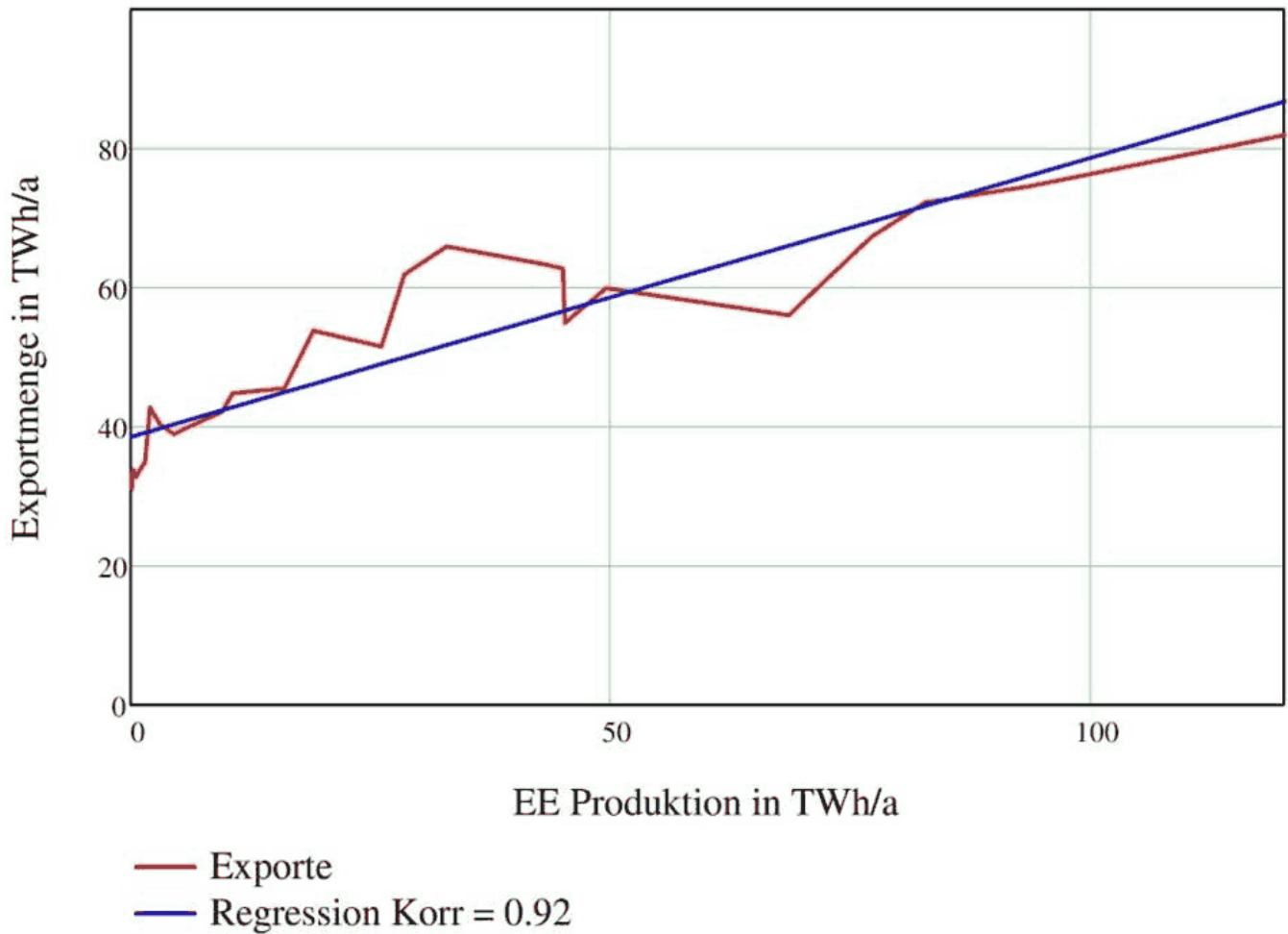
Abbildung 6: Ansteigender Stromexport verursacht durch volatile Stromproduktion aus Wind und Solarenergie
