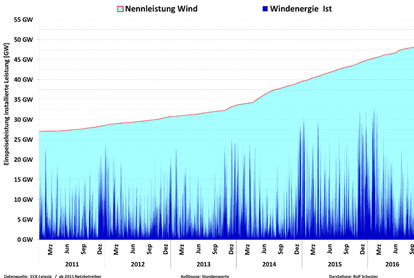
Abbildung 3: Windstromproduktion Deutschland von 2011 bis 2016
