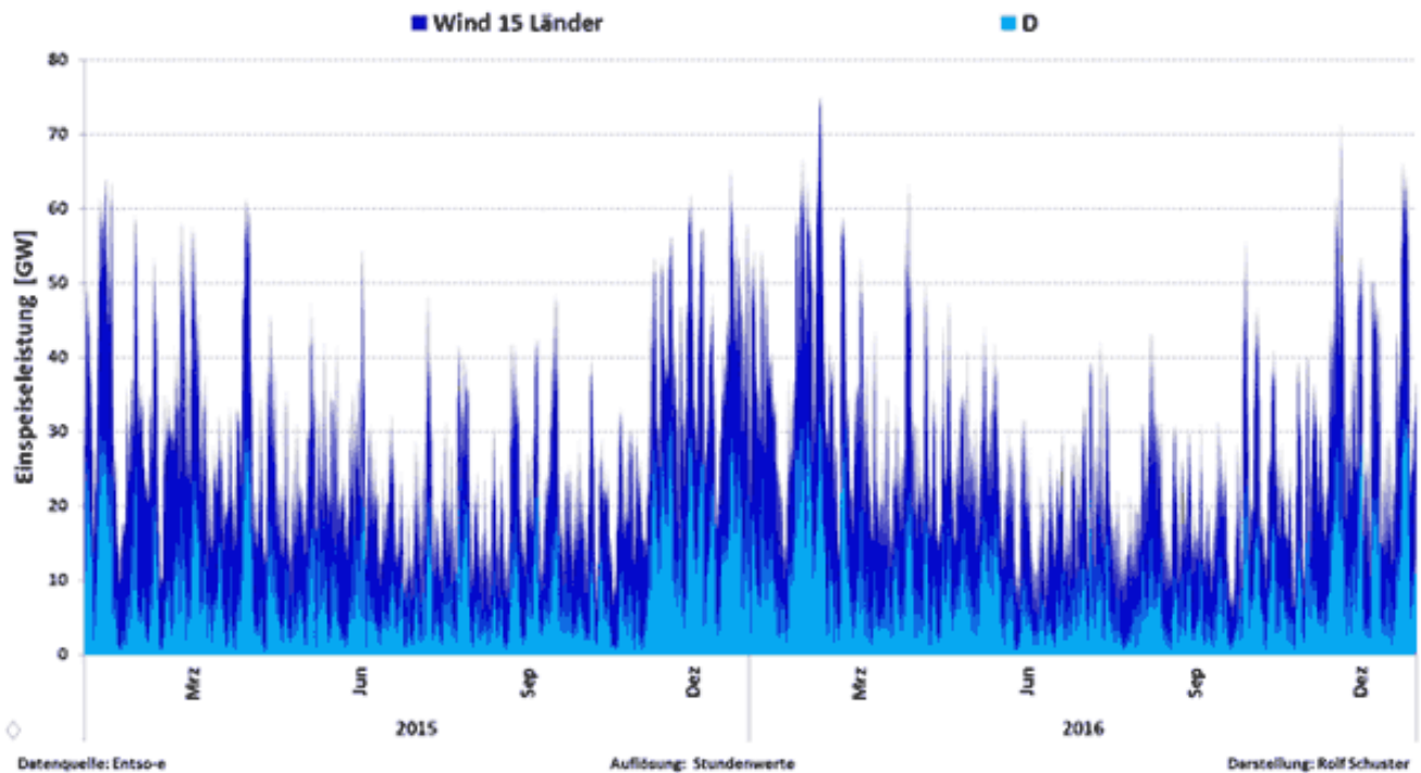
Abbildung 4: Windstromproduktion von 15 europäischen Ländern
